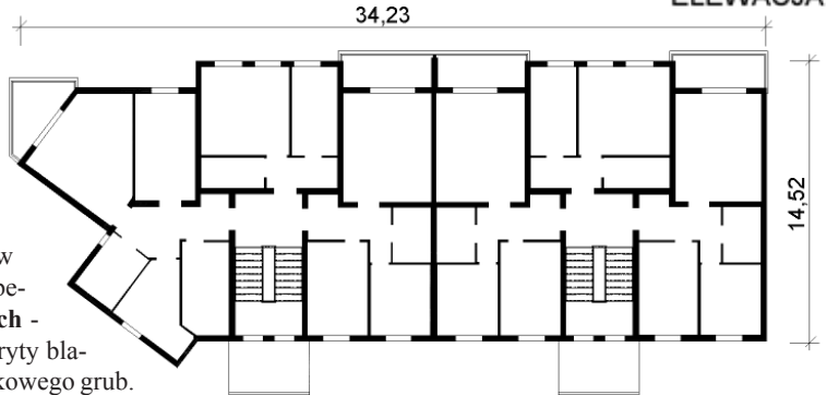
RZUT PIĘTRA
