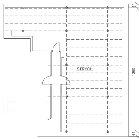
Rzut poddasza
